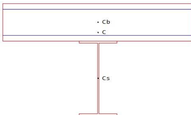
Рис. 1. Составное сечение балки с верхним расположением плиты
