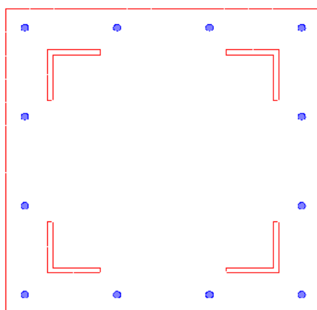
Рис.12. Сечение с жесткой арматурой из уголков
