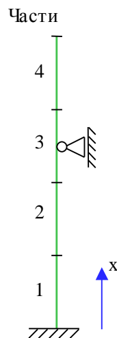
Рис. 1. Расчетная схема
