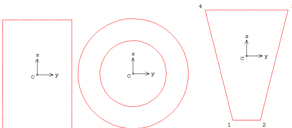
Рис. 1. Виды сечений
