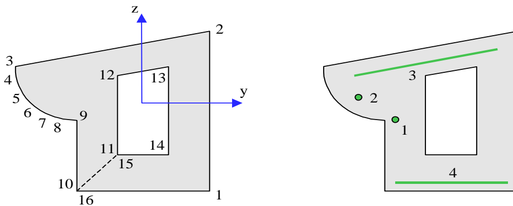
Рис. 4. Сечения
