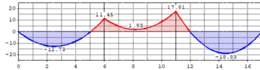
Изгибающий момент M_z , [кНм]
