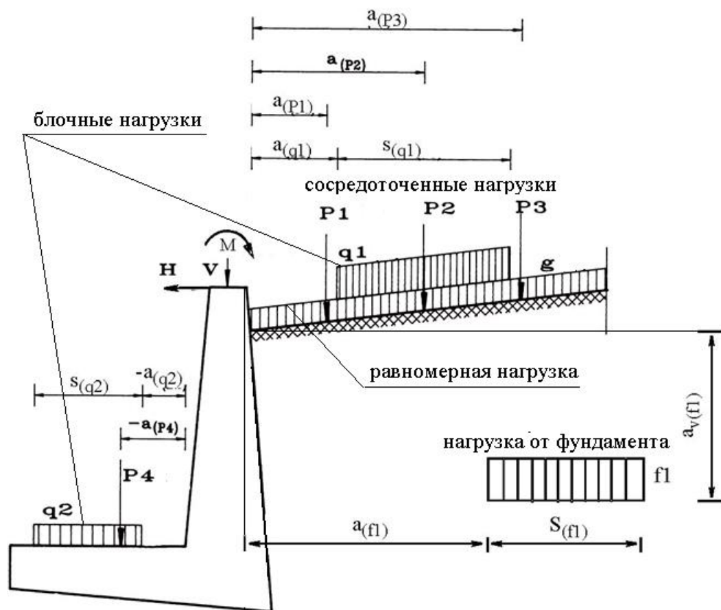
Рисунок 2: Нагрузки
